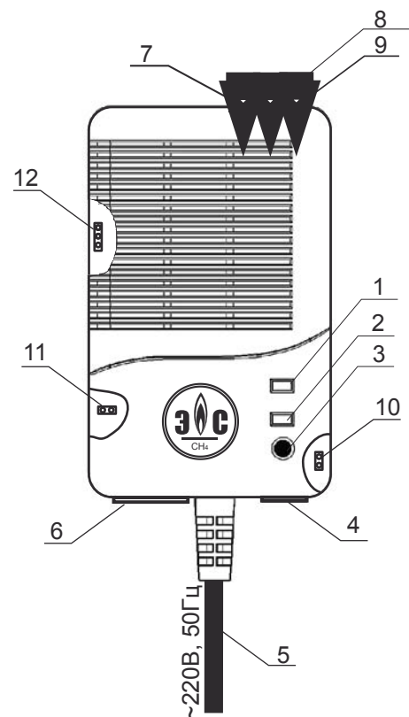
Сигнализатор СЗЦ-1(2)-0.Р.С.
