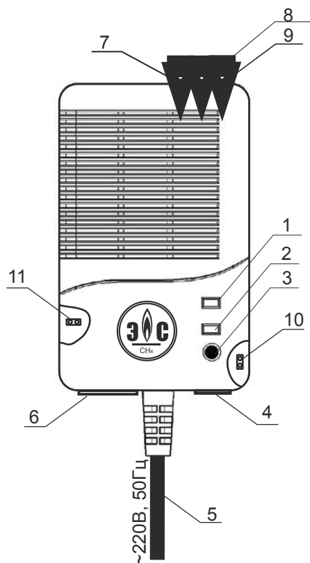
Сигнализатор СЗЦ-1(2)-0
