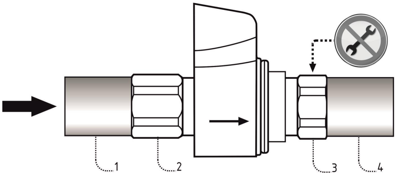
Рисунок В1 – схема установки клапана на трубопровод
