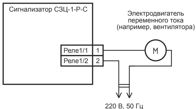
Подключение дополнительных устройств к сигнализаторам СЗЦ-...-Р-С
